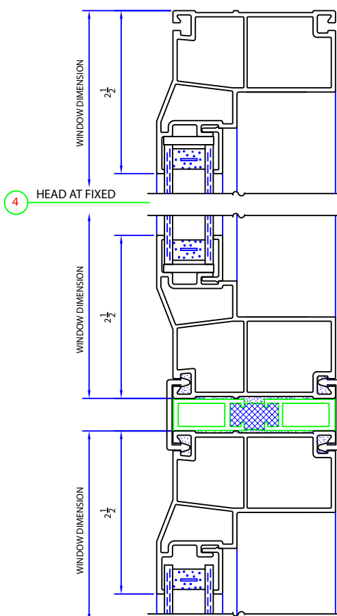
3 TYP. MULLION
